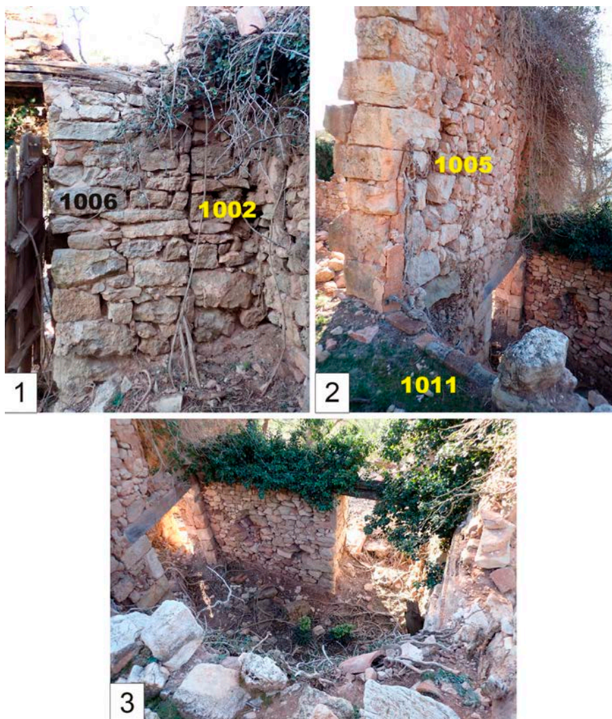
Figura 10| Sector 2, àmbit A: 1. Parament interior del mur 1002 i brancal NO de la porta 1006. 2. Restes de la porta 1011 a nivell de primera planta en el mur de tancament NO (1004). 3. Visió zenital de l'àmbit A on s'observen les portes 1008 i 1003.
