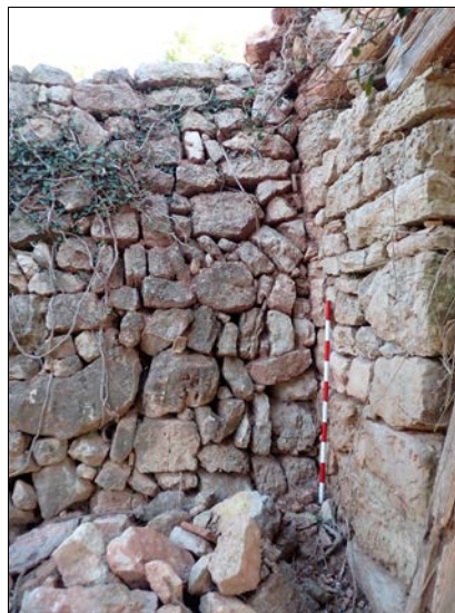
Foto 37. Punt d'adossament del marge 1001 contra el mur de façana de l'àmbit B (1010).
