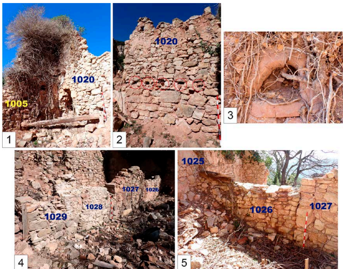
Figura 7| Sector 1, àmbit C: 1. Cantonada SO de l'àmbit C amb la unió dels murs 1020 i 1005. 2. Mur 1020 amb les marques de la inserció del forjat de la primera planta. 3. Fornícula 1014 en el mur 1005. 4. Tancament SE de l'àmbit C amb els elements estructurals documentats (vista des de l'interior de l'àmbit D). 5. Mur 1026 i biga associada.
