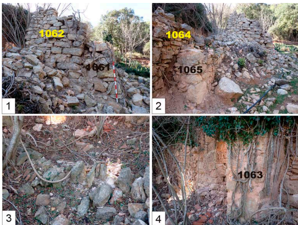
Figura 14| Sector 3, àmbits E i F: 1. Mur de tancament SE de l'àmbit K reforçat per la contraparet 1061. 2. Mur de reforç 1065 que es recolza al mur de tancament NE 1064. 3. Marge amb lloses verticals (1070) present dins l'àmbit K. 4. Contrafort 1063 que s'adossa al mur 1015.
