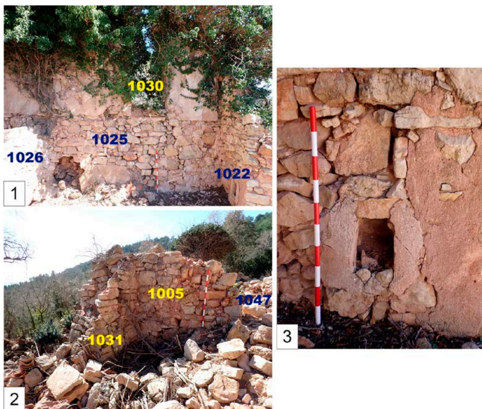
Figura 8| Sector 1, àmbit D: 1. Visió frontal del mur 1025, amb porta a nivell de primera planta (1030). 2. Cantonada SO de l'àmbit amb els murs 1005 i 1031. 3. Detall de l'orifici rectangular 1022 present al mur 1022.
